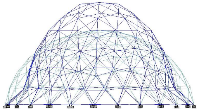
Fig. 10 b).Modal shape 2
